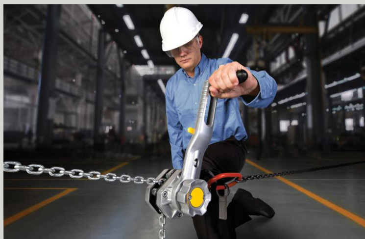
PÁKOVÉ KLADKOSTROJE
