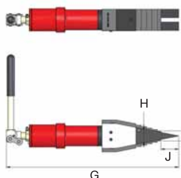
SJS10 M Vysunuto
