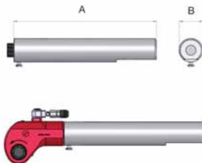
TWS-N opatřené prodlouženým reakčním ramenem
