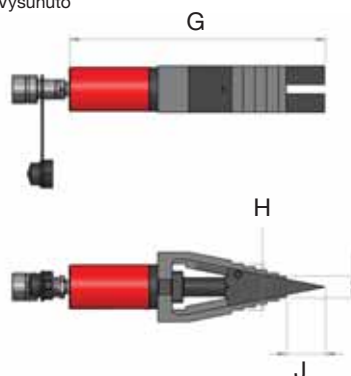
SJS10 M Vysunuto
