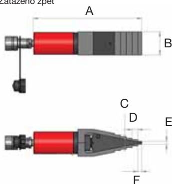
SJS10M Zataženo zpět
