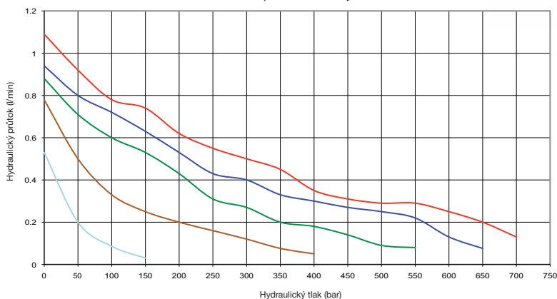
Graf průtok / tlak oleje
